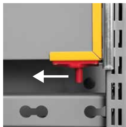
Einhändiges Öffnen des Regals Opening shelf-system with one hand
