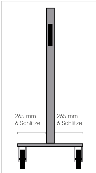
WAGEN SMART 102 - 103
