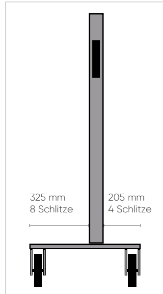
WAGEN SMART 102
