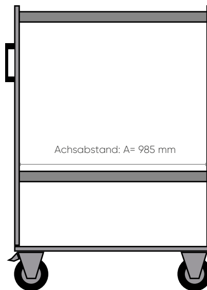
WAGEN SMART 101 - 102 - 103
