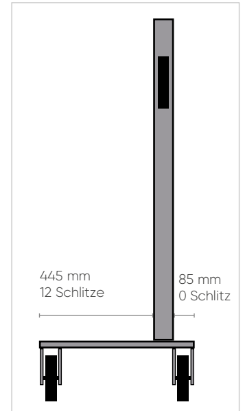
WAGEN SMART 101 - 102
