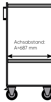
WAGEN SMART 073
