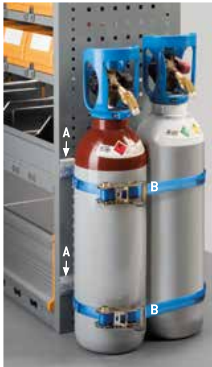
Beispiel mit 2 ART. NR. / ITEM NO. V18029 03 2 ART. NR. / ITEM NO. V22868 Example with 2 ART. NR. / ITEM NO. V18029 03 2 ART. NR. / ITEM NO. V22868
